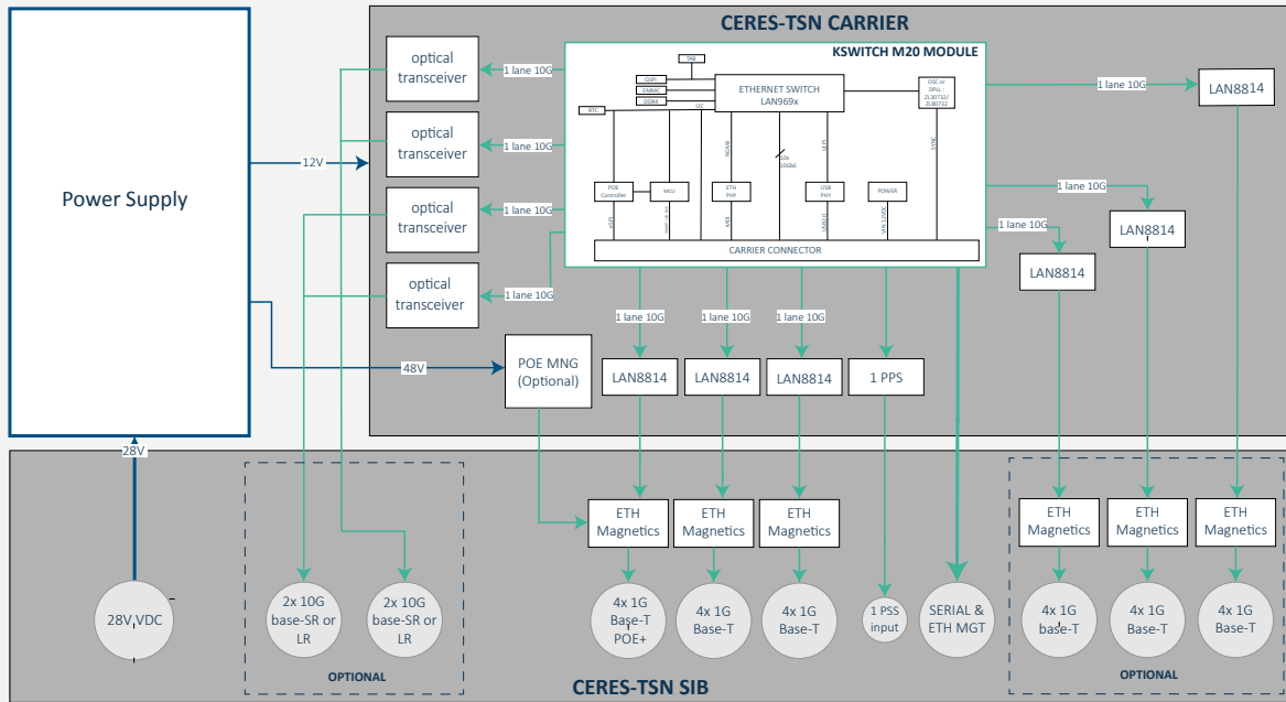
CERES-TSN-2404 & CERES-TSN-1202
